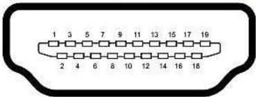
Piedinatura
