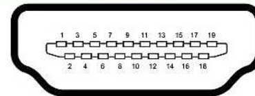
Piedinatura
